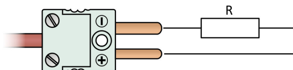
Obrázek 13T.17: RTD v dvou vodičovém zapojení s miniaturním konektorem
